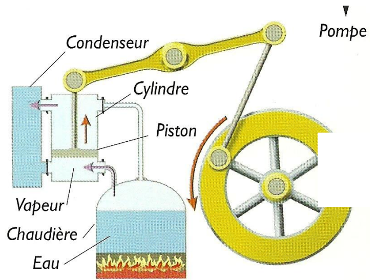
Doc. 3 Machine à vapeur de James Watt
